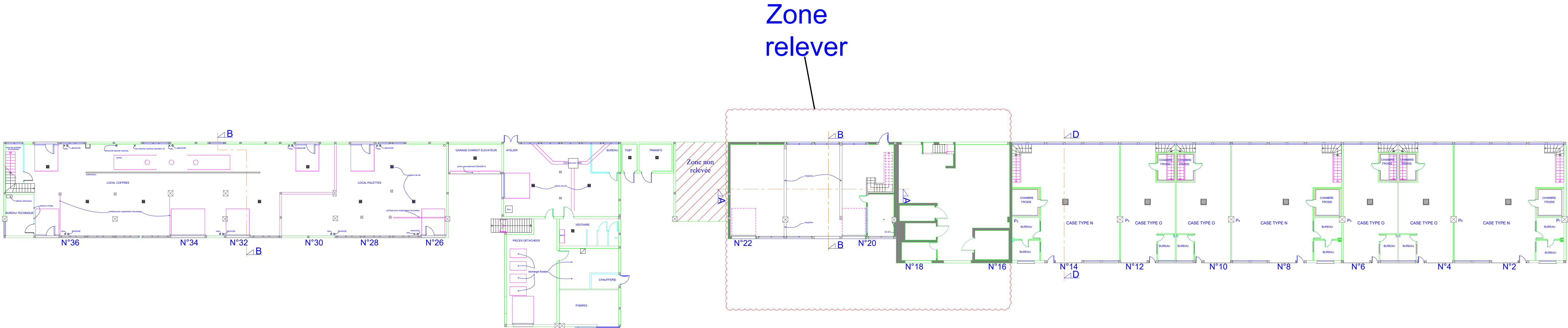
PLAN REZ DE CHAUSSEE LOCAL COFFRES ET PALETTE DU N°36 AU N°26 PLAN REZ DE CHAUSSEE SERVICE DES PECHES PLAN REZ DE CHAUSSEE DU N°22 AU N°20 PLAN REZ DE CHAUSSEE N°18 AU N°16 PLAN REZ DE CHAUSSEE CASES DE MAREYEURS DE TYPE "N","O" N°14 AU N°2
